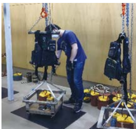
荷重試験 吊下げ部の強度試験 大人用 880N(約90kg)/5分。 小児用、幼児用 580N(約59kg)/5分
